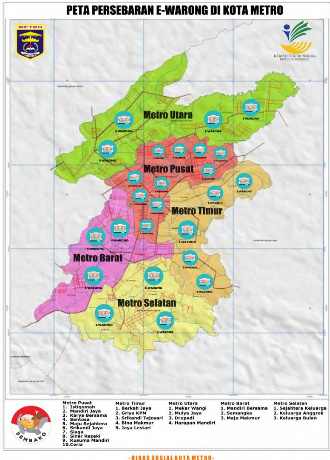
Gambar 6.1. PETA PERSEBARAN E- WARONG DI KOTA METRO TAHUN 2023
